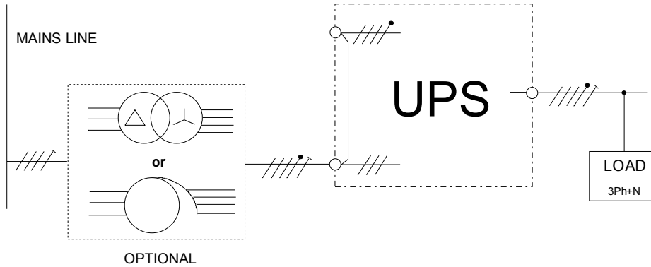
- Одиночная линия питания без нейтрали -
